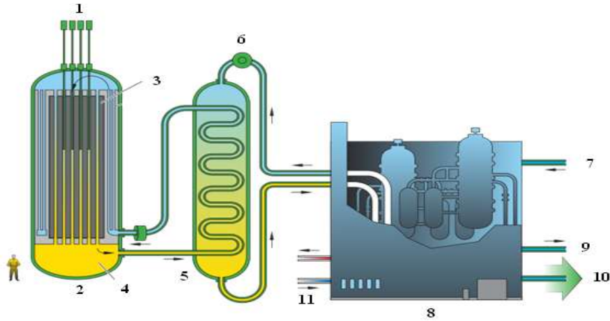
الشكل (1) المفاعل الذي يعمل عند درجة حرارة مرتفعة جداً
