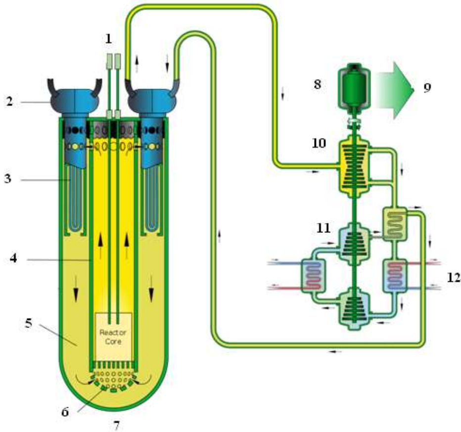
الشكل (6) المفاعل السريع المبرد بالرصاص
