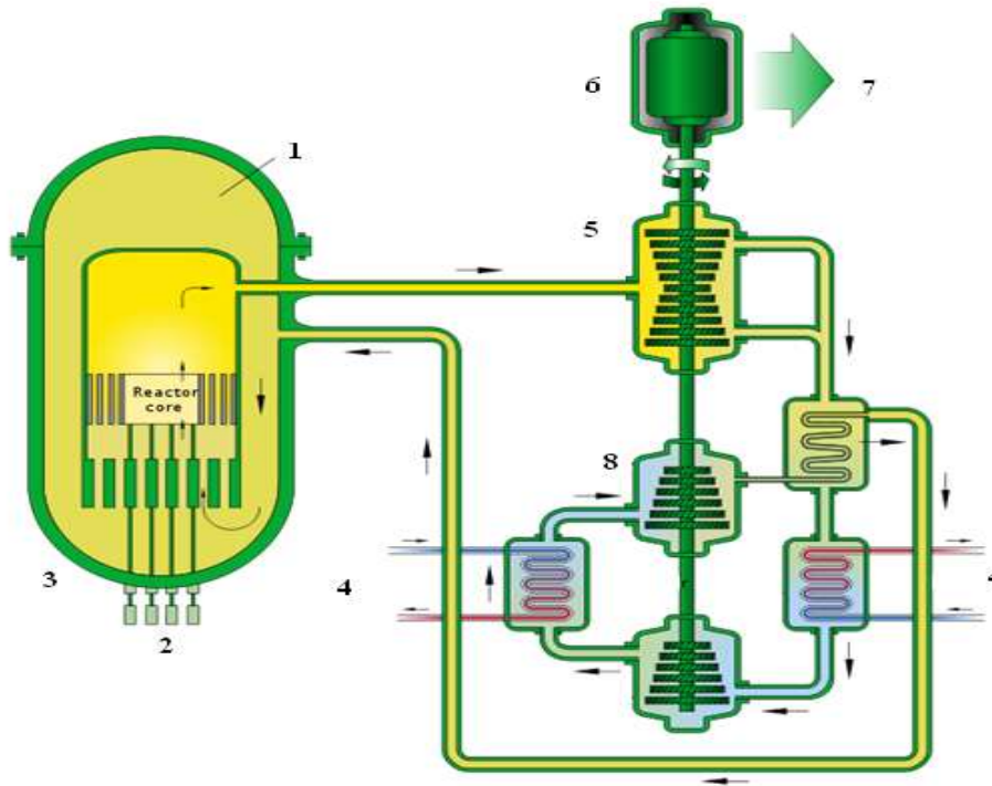
الشكل (4) المفاعل السريع المبرد بالغاز
