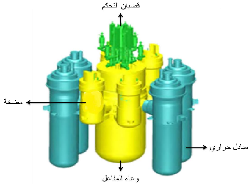
الشكل (1) صورته توضيحية لأجزاء المفاعل KLT-40S
