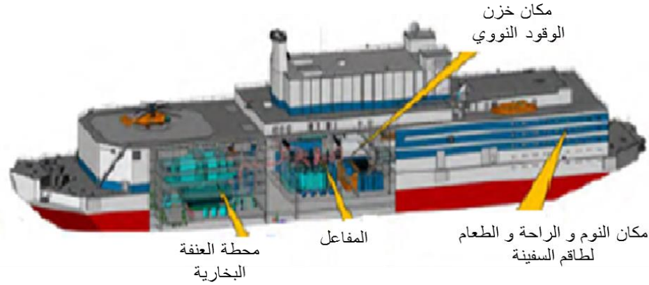
الشكل (2) صورته توضيحية للمحطة النووية العائمة على مياه البحر (FNPP) والتي يتم تشغيلها بالمفاعل النووي KLT-40S.
